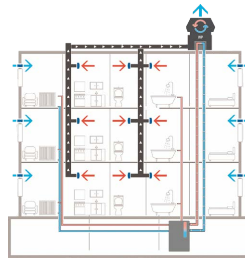
Die Aereco AWN ermöglicht eine ganzjährige Wärmebereitstellung (Wärmerückgewinnung und -erzeugung) und ist damit am Markt nahezu einzigartig © Aereco
